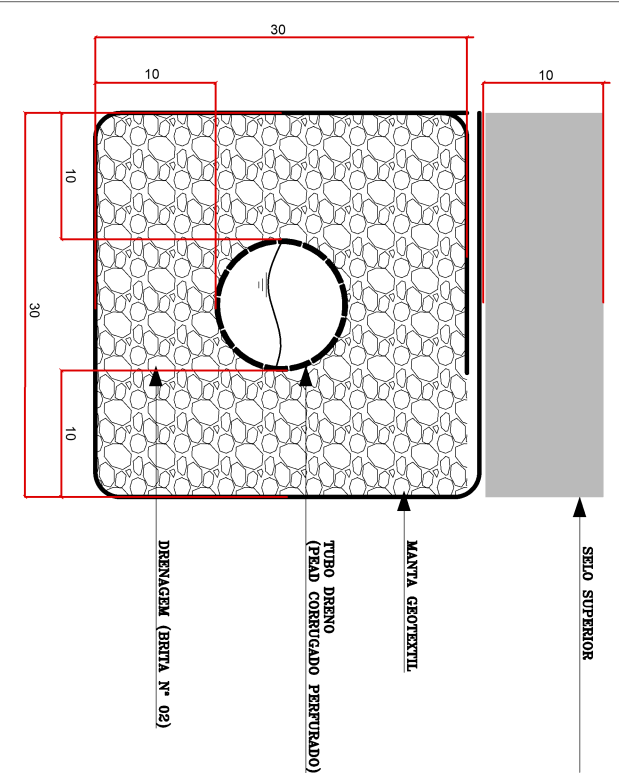
DETALHE DRENAGEM S/ ESCALA
